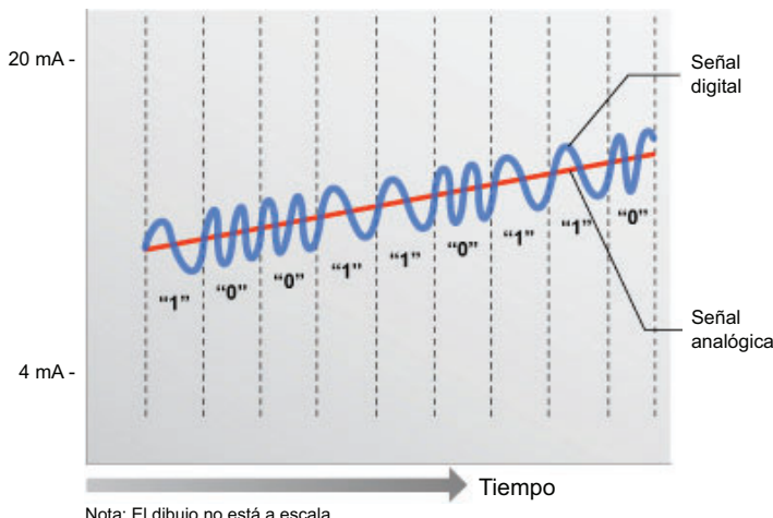
Codificación por cambio de frecuencia Digital sobre analógico
