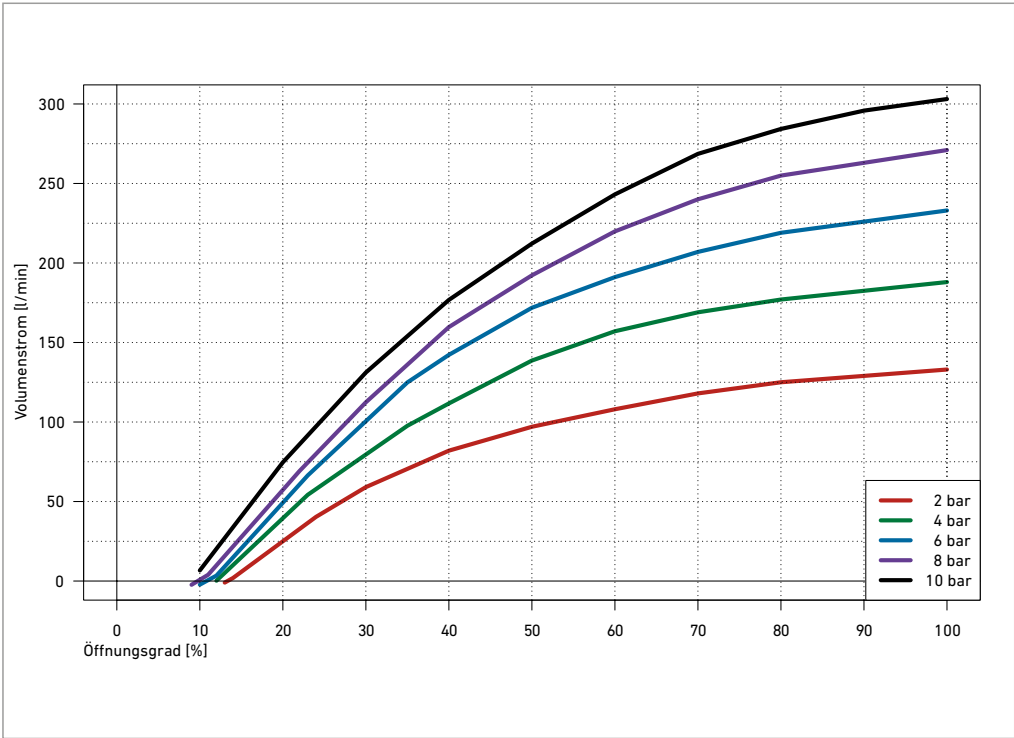
Spüleistung DN20
