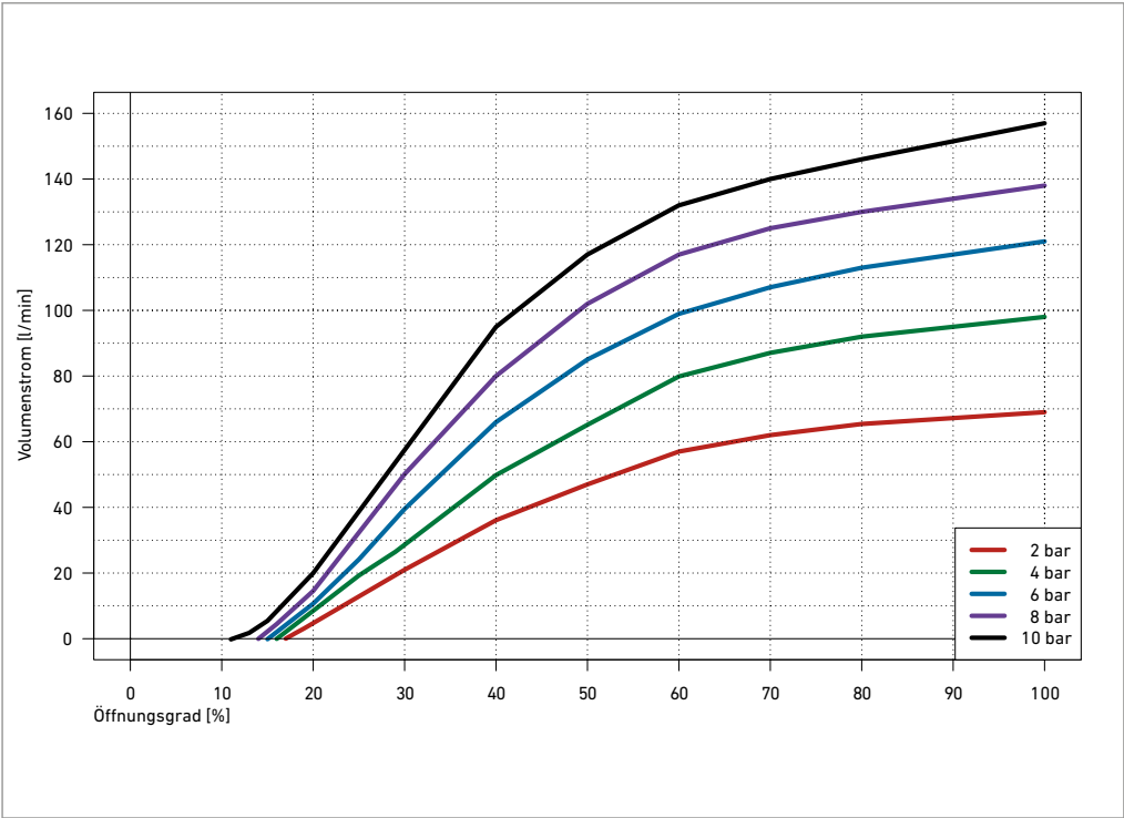
Spüleistung DN15
